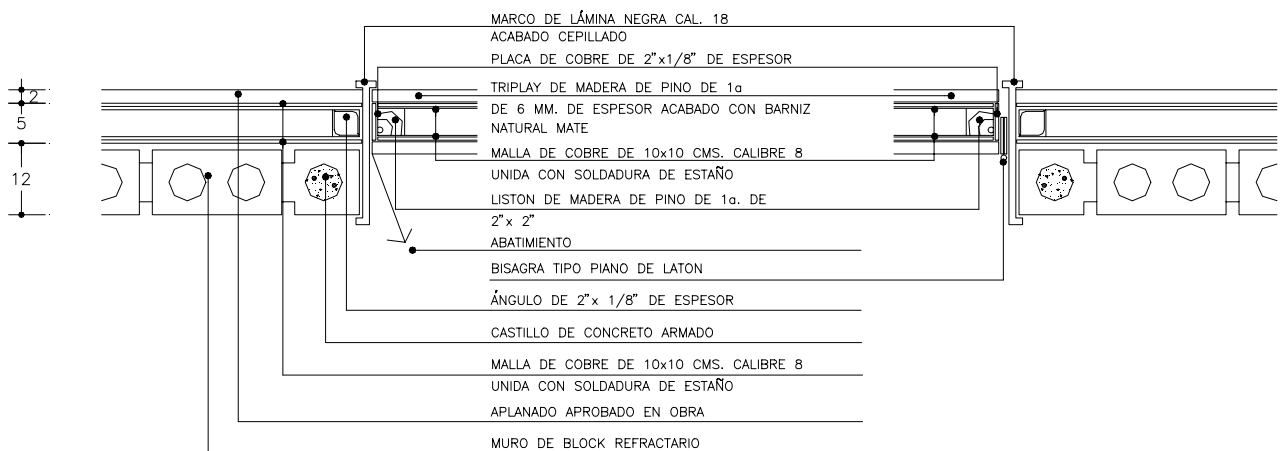
DETALLE PUERTA DT-7
