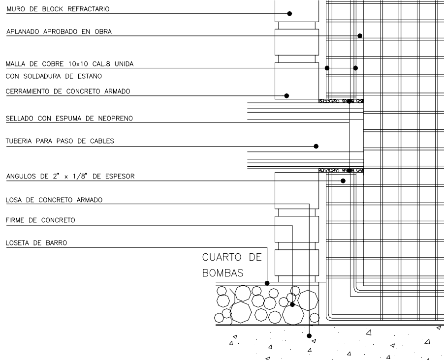
DETALLE PASO DE CABLES DT-6
