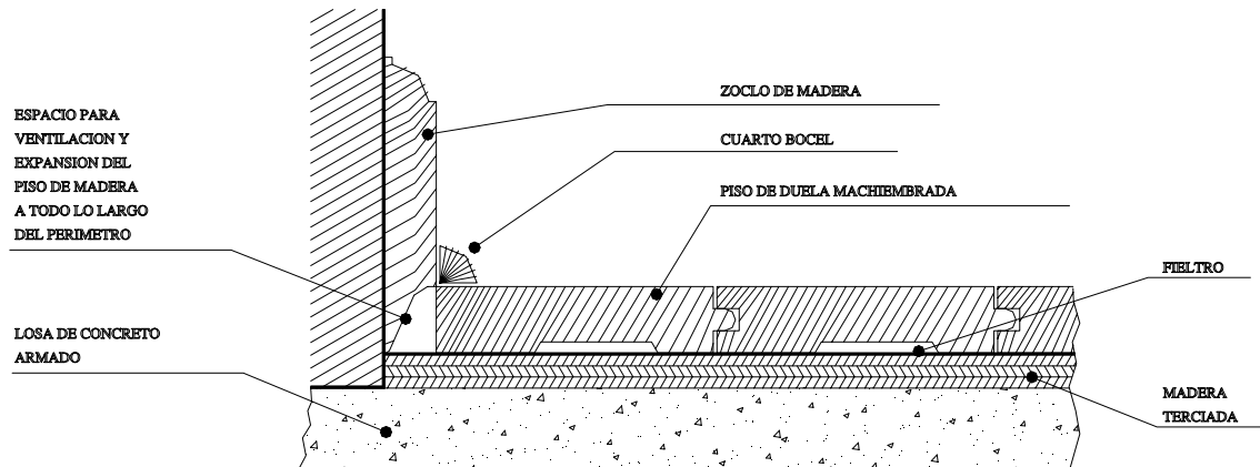
DETALLE DE VENTILACION Y EXPANSION
