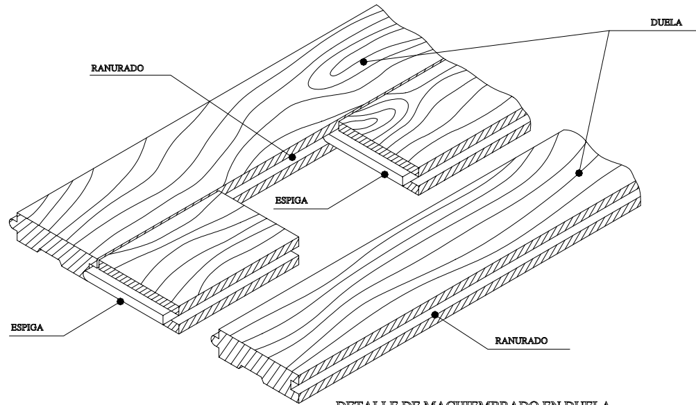
DETALLE DE MACHIEMBRADO EN DUELA
