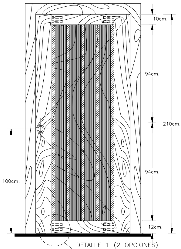
ALZADO PUERTA ENTABLERADA
